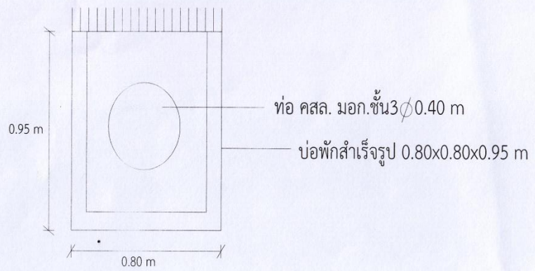
รูปตัด A
