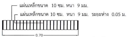
รูปตัด ๑ ฝาปิดตะแกรงเหล็ก
