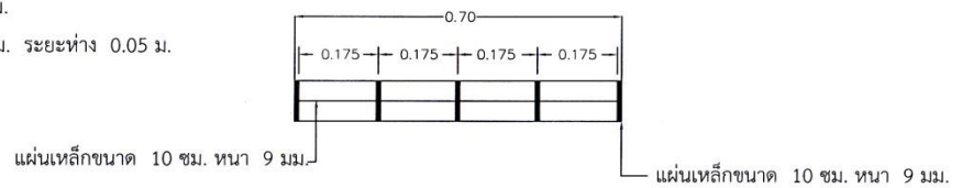
รูปตัด ๒ ฝาปิดตะแกรงเหล็ก
