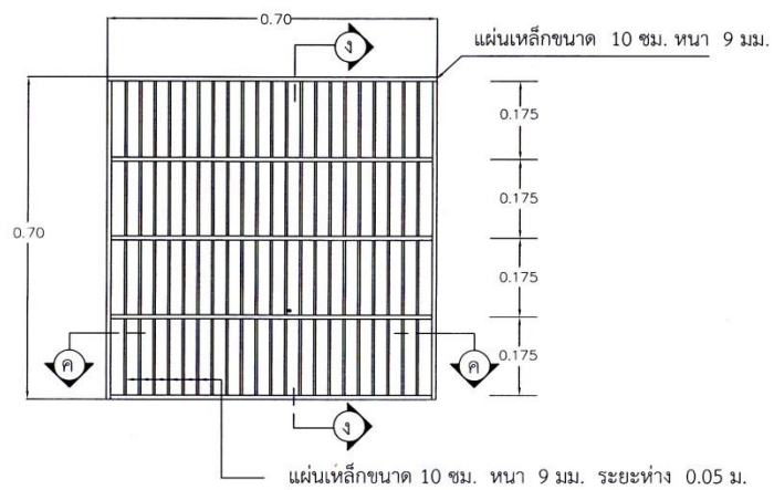
แปลน ฝาปิดบ่อพักตะแกรงเหล็ก
