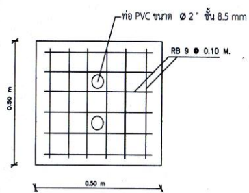
รายละเอียดเหล็กเสริมฝาปิดรางน้ำ
