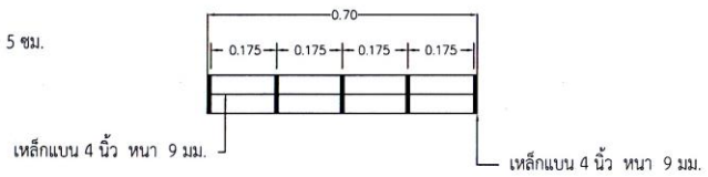
รูปตัด ข ฝ่าปิดตะแกรงเหล็ก
