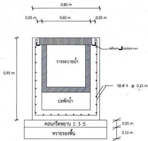
รูปตัด ก บ่อพักน้ำ ค.ส.ล.
