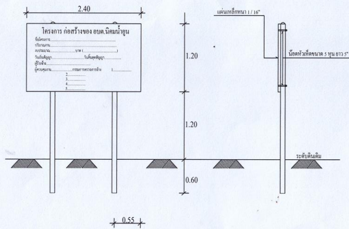
รูปด้านหน้า
