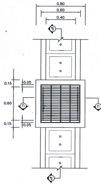
แปลน บ่อพักน้ำและรางระบายน้ำ
