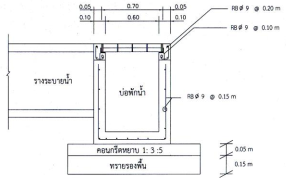
รูปตัด ข บ่อพักน้ำ ค.ส.ล.
