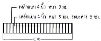
รูปตัด ก ฝ่าปิดตะแกรงเหล็ก
