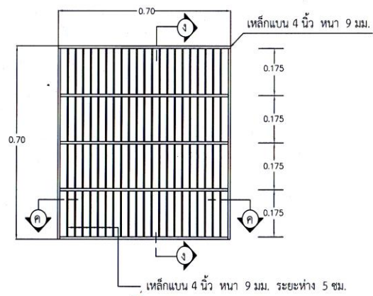
แปลน ฝ่าปิดบ่อพักตะแกรงเหล็ก
