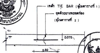
LONGITUDINAL JOINT
