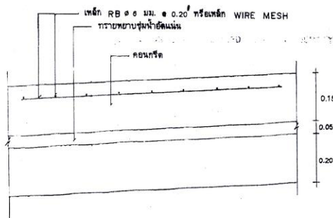
รายละเอียดคานคอนกรีตเสริมเหล็ก
