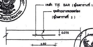
LONGITUDINAL JOINT
