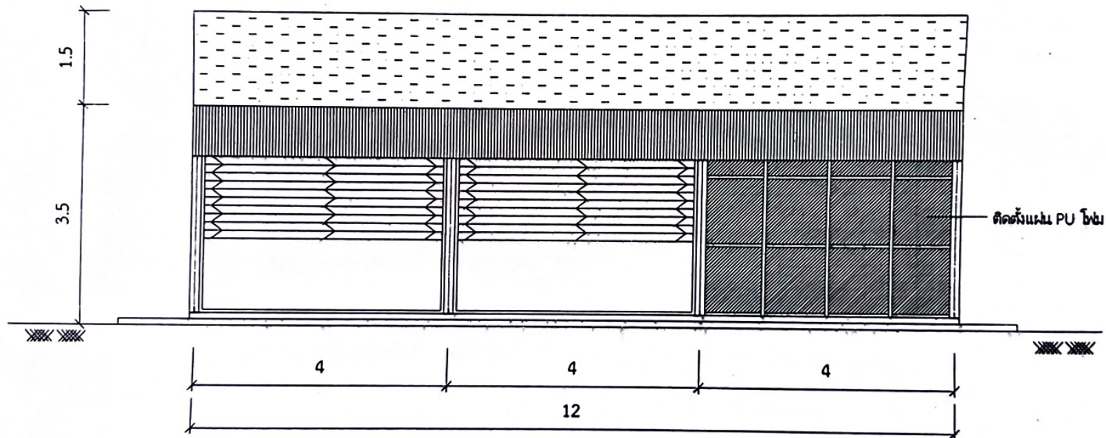
รูปด้าน A
