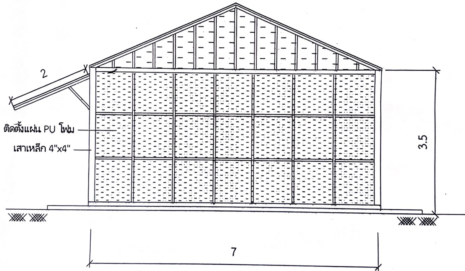
รูปตัด D
