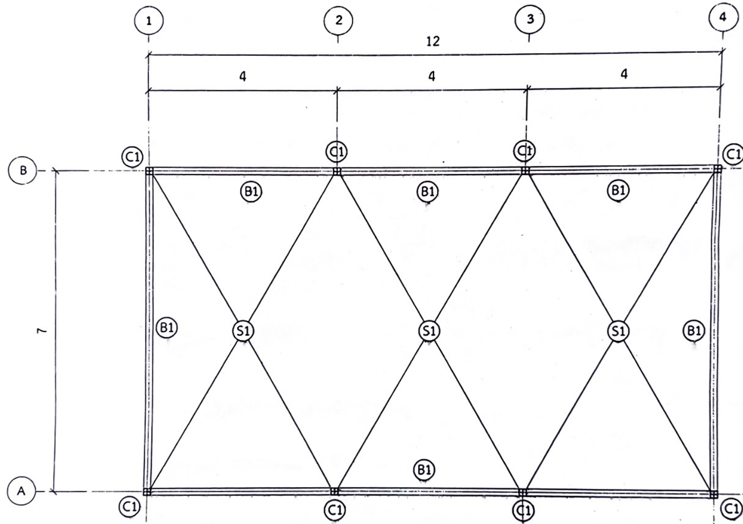
แปลน เสา คาน พื้น
