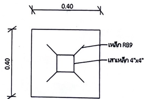
แปลนฐานราก
