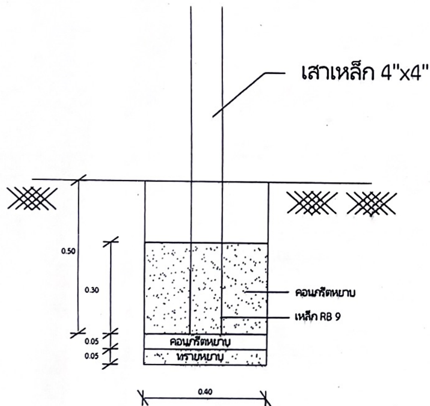
รูปตัดฐานราก
