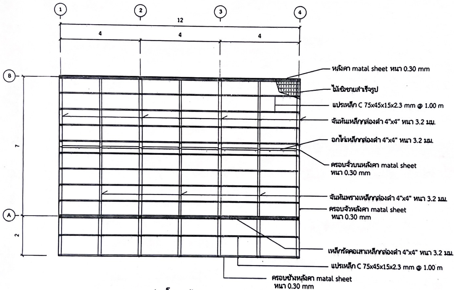
แปลนโครงหลังคา
