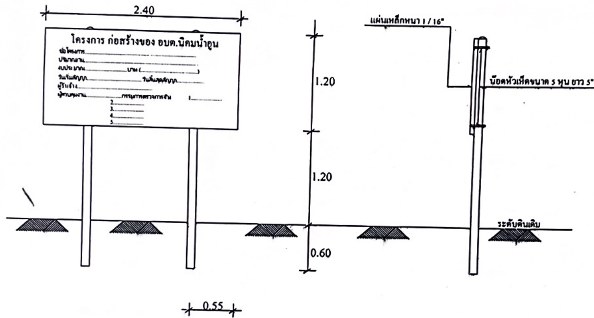
รูปด้านหน้า
