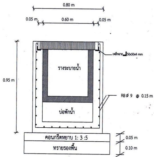
รูปตัด ก) บ่อพักน้ำ ค.ส.ล.
