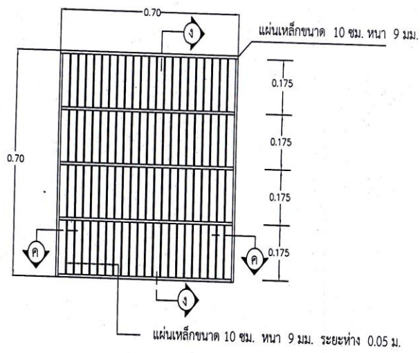
แปลน ฝาปิดบ่อพักตะแกรงเหล็ก
