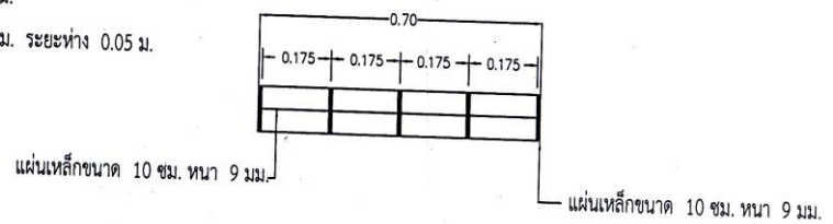
รูปตัด ๒ ฝาปิดตะแกรงเหล็ก
