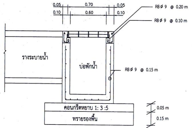
รูปตัด ข) บ่อพักน้ำ ค.ส.ล.
