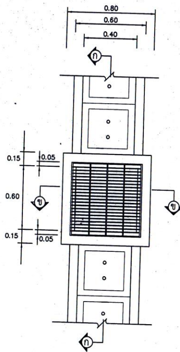
แปลน บ่อพักน้ำและวางระบายน้ำ
