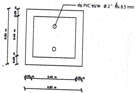
ฝาปิดรางระบายน้ำ
