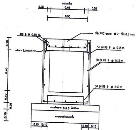
รายละเอียดเหล็กเสริมรางน้ำ
