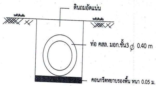
รูปตัด B
