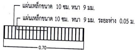
รูปตัด ๑ ฝาปิดตะแกรงเหล็ก
