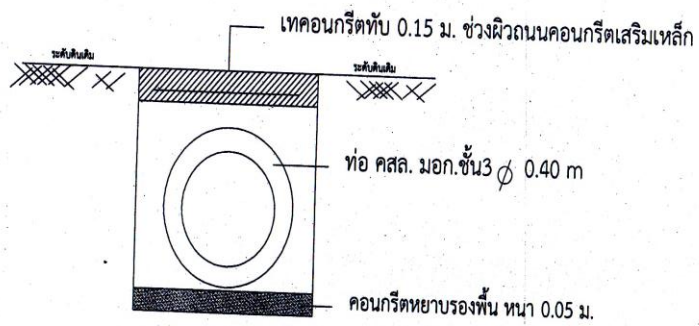
รูปตัด A
