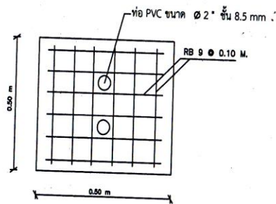
รายละเอียดเหล็กเสริมฝาปิดรางน้ำ
